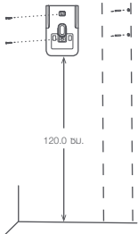
การติดตั้งตัวติดตั้งบนผนังสำหรับเครื่องดูดฝุ่น
