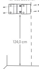
Installation der Wandhalterung für das Zubehör
