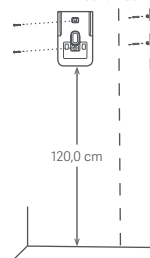
Montaż uchwyty ścienne na odkurzac
