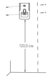
Встановлення настінного кріплення для аксесуарів
