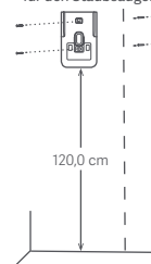
Installation der Wandhalterung für den Staubsauger
