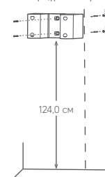
Шаңсорғышты қабырғаға бекіту құралын орнату
