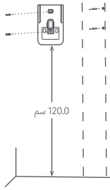
التثبيت حامل الحائط للمكنسة الكهربائية
