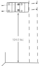
การติดตั้งตัวติดตั้งบนผนังสำหรับอุปกรณ์เสริม
