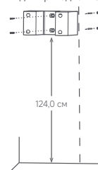
Монтаж настенного крепления для принадлежностей
