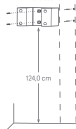
Montaż uchwyty ścienne na akcesoria
