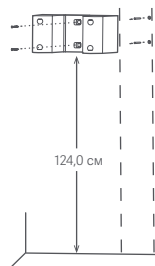
Встановлення настінного кріплення для пилососа
